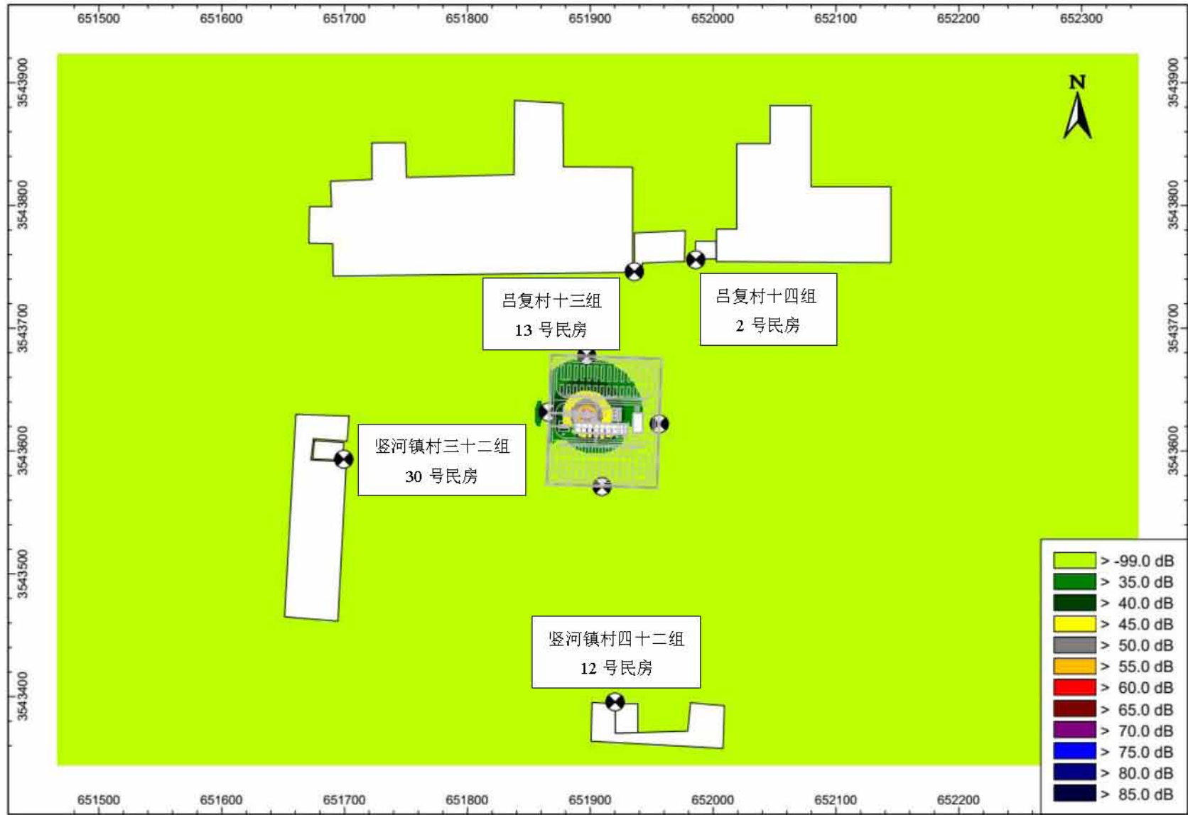
图 4.8-2 本工程建成运行噪声贡献值等声级线分布图（预测点高度为地面上方 1.2m）
