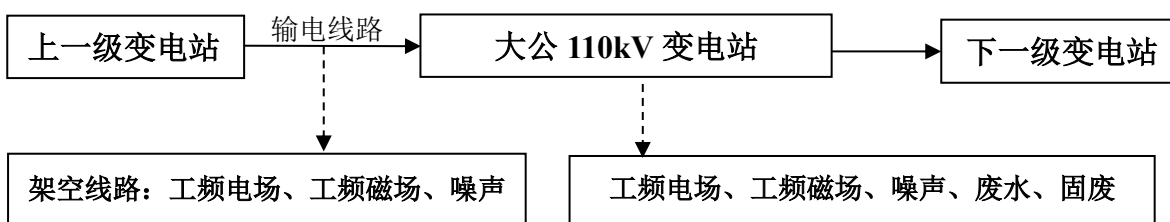
图 1 南通大公 110kV 输变电工程工艺流程及产污环节示意图
